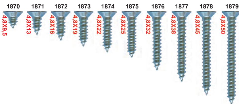
CABEÇA CHATA/PHILLIPS
